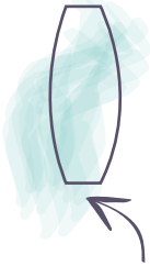
LENTE BICONVESSA
